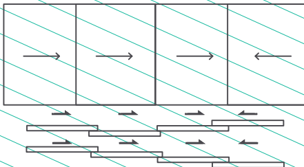
Cancel corredizo de cuatro hojas No. de rieles: 4
