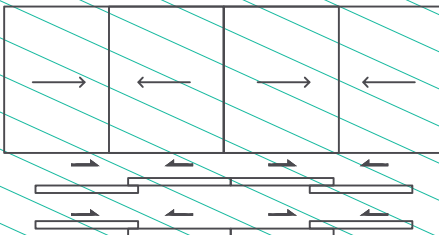
Cancel corredizo de cuatro hojas No. de rieles: 2
