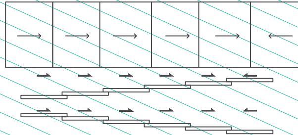
Cancel corredizo de 6 hojas No. de rieles: 6
